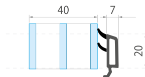
044 ШТАПІК
