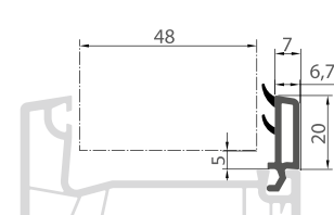
141 ШТАПІК
