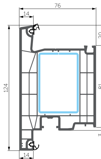
138 СТУЛКА
