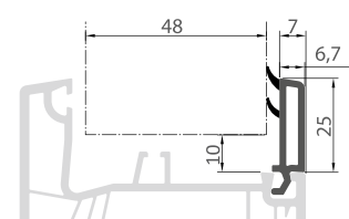
132 ШТАПІК
