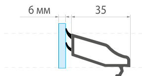
004 ШТАПІК
