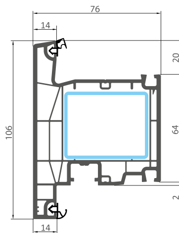
044 ШТАПІК
