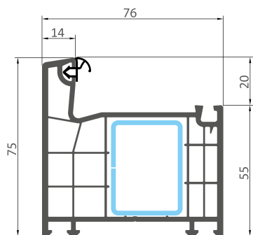
139 ІМПОСТ
