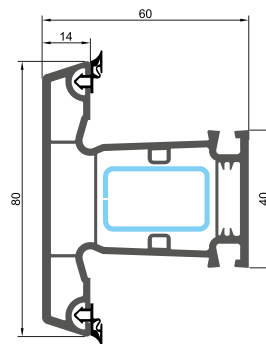
044 ШТАПІК
