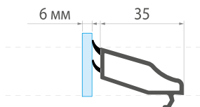
004 ШТАПІК
