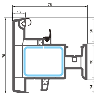
130 ШТУЛЬП
