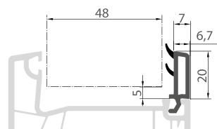
044 ШТАПІК
