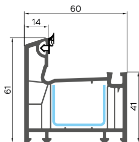
086 РАМА
