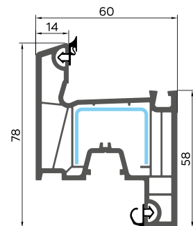
087 СТУЛКА
