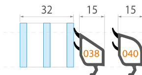
038, 040 ШТАПІК
