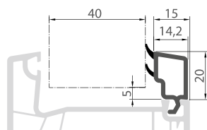
004 ШТАПІК
