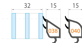
038, 040 ШТАПІК
