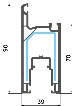
099 СТУЛКА
