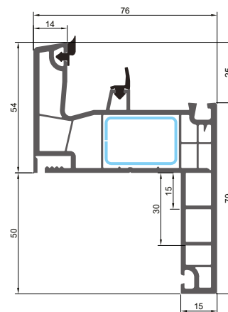
129 РАМА
