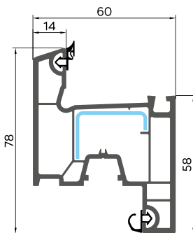
039 СТУЛКА
