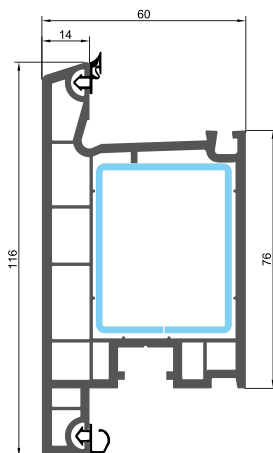
018 ІМПОСТ
