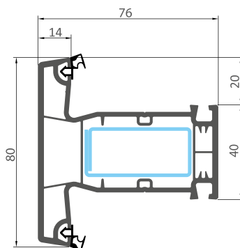
145 ІМПОСТ
