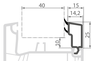
131 ШТАПІК
