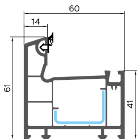
017 РАМА
