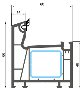
001 РАМА
