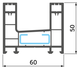
094 РАМА
