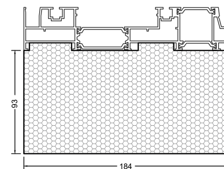
Рама 2-рейкова
