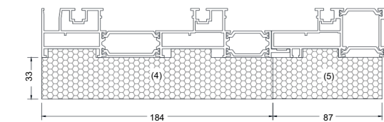
Рама 3-рейкова
