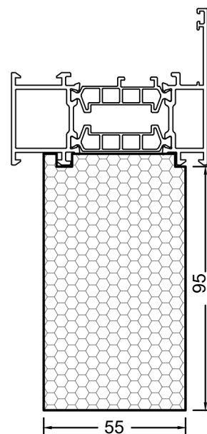
Рама віконна W76
