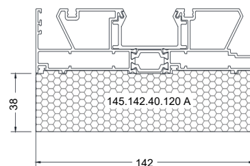
Рама 2-рейкова WS142
