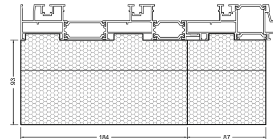
Рама 3-рейкова
