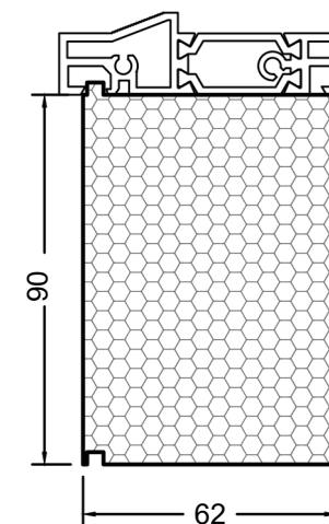
Поріг 7521 для PE78N
