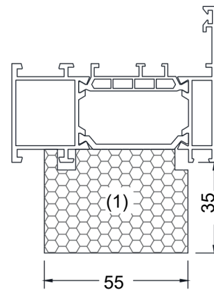
Рама віконна PE78N
