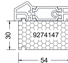
Поріг 7522 для PE78N
