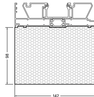
Рама 2-рейкова WS142
