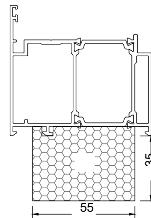
Рама дверна W76
