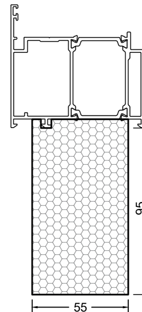
Рама дверна W76
