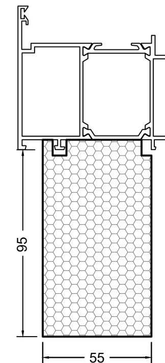
Рама дверна PE78N
