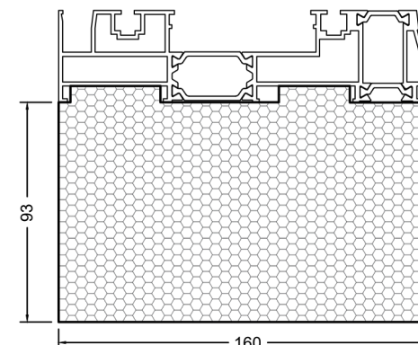
Рама монорейкова та 2-рейкова
