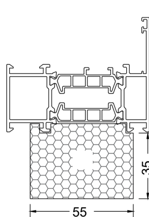
Рама віконна W76
