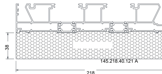
Рама 3-рейкова WS142
