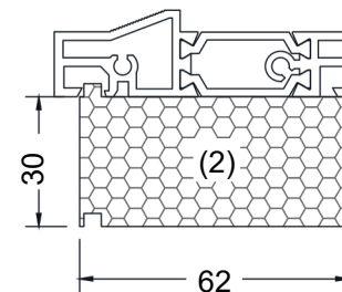
Поріг 7521 для PE78N
