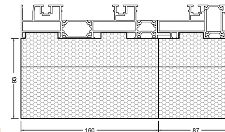
Рама 3-рейкова
