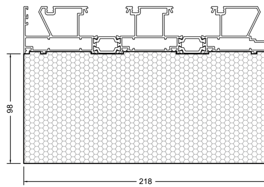
Рама 3-рейкова WS142
